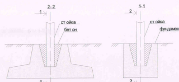
Рис. 1 Закрепление опор знаков в фундаменте
