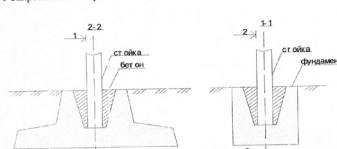
Рис. 1 Закрепление опор знаков в фундаменте
